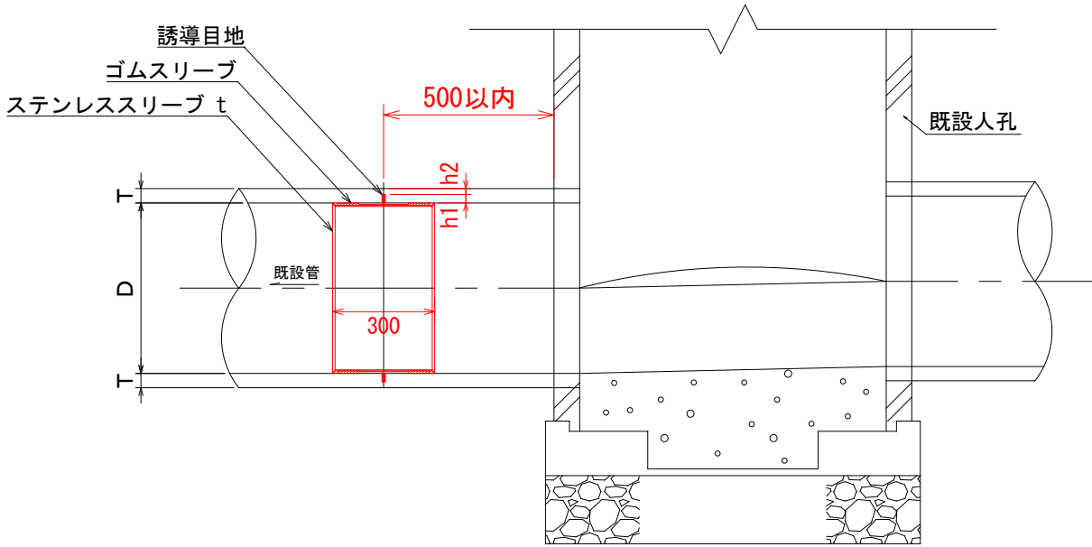
外圧管 寸法表
