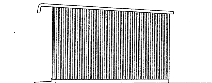
3通 立面図
