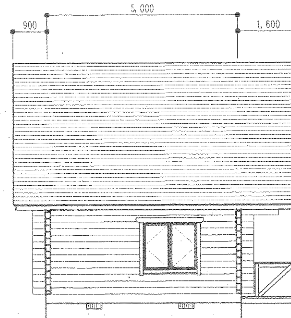
B 立面図 S=1/100
