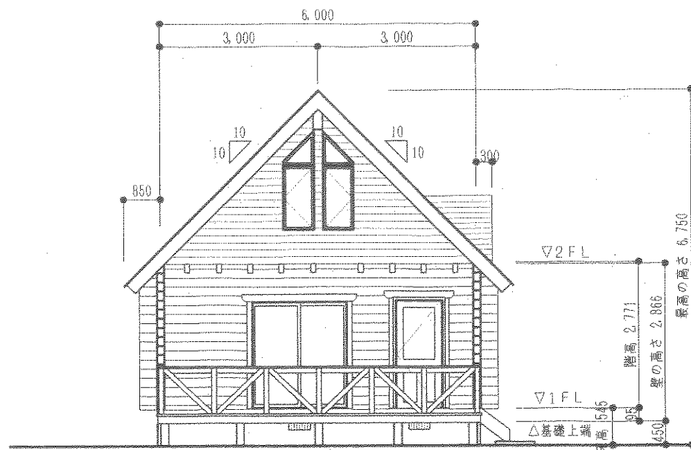
A 立面図 S=1/100
