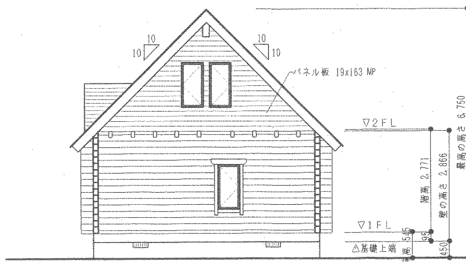
C 立面図 S=1/100
